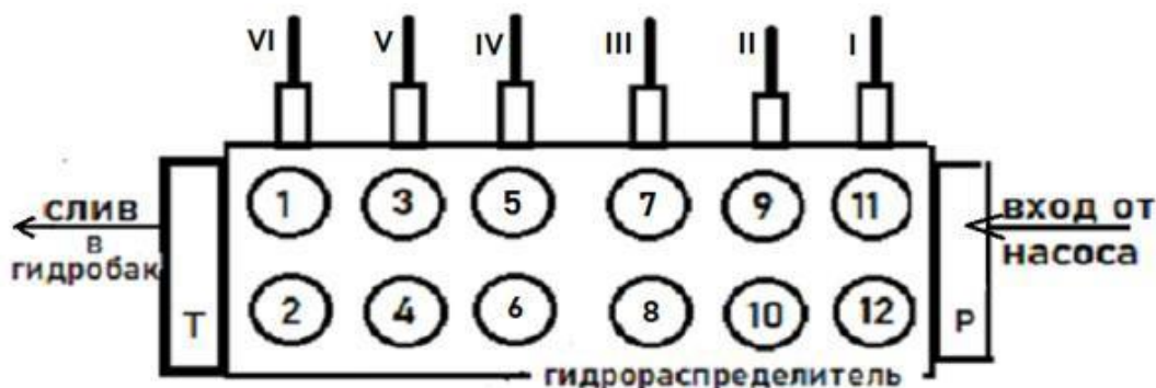
Вид на места присоединения РВД от гидроцилиндров к гидрораспределителю (со стороны стрелы)
